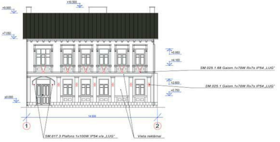
FASĀDE 1-2 M1:100
