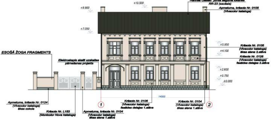
FASĀDE 1-2 M1:100
